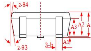
侧视图
