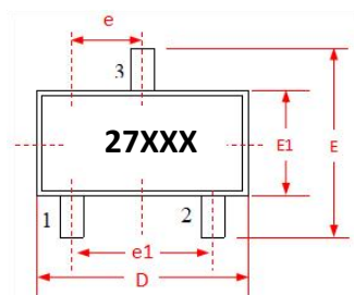
俯视图
