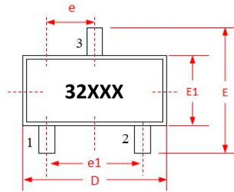
俯视图
