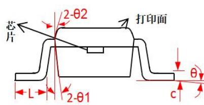
侧视图
